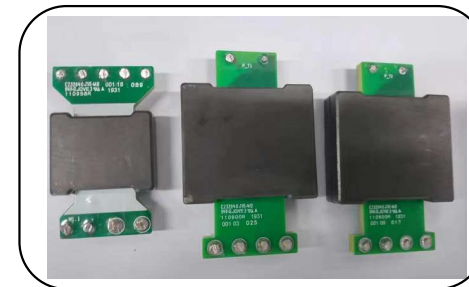
扁平设计电感及PCB集成变压器
