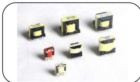
EE/EF/EI /EP/PQ 型高频变压器
