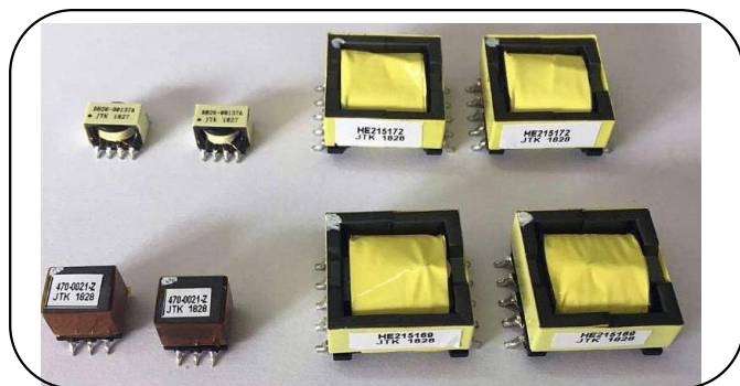
SMD 贴片电感、变压器
