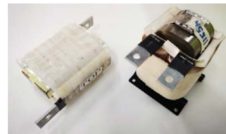
铜滤波绕制，大电流 焊接加工车间
